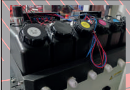
SISTEMA BULK INK CON SENSOR DE NIVEL DE TINTA
