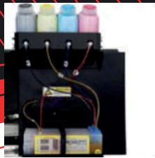
Sistema Bulk Ink
